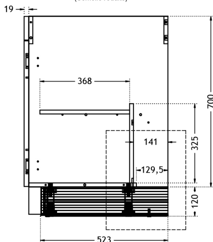
VUE DE DROITE (Semelle réduite)
