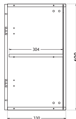
VUE DE DROITE
