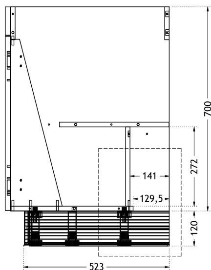
VUE DE DROITE (Semelle réduite)
